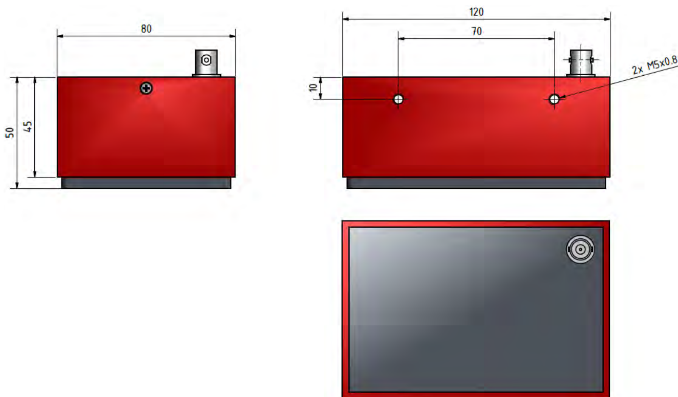
Fig. 4: Stator antenna A8f_PCM
