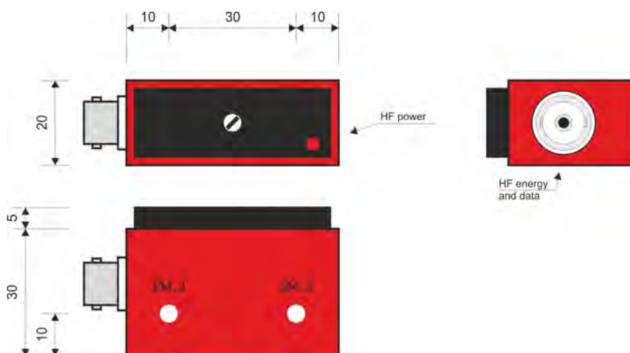
Fig. 4: Stator antenna A8a_PCM
